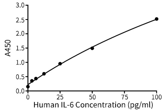
图3. Human IL-6 ELISA Kit (High-sensitive)的标准曲线。实测数据会因实验条件、检测仪器等的不同而存在差异，图中数据仅供参考。
